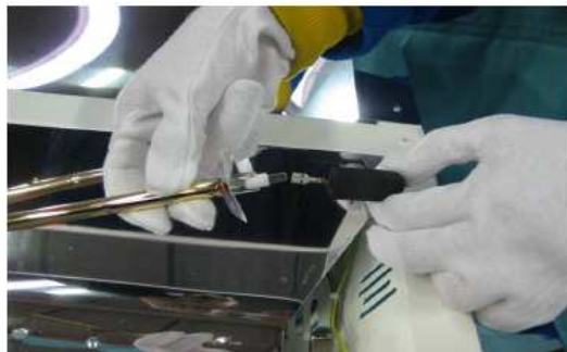
4. DIE BEIDEN SILIKONDICHTUNGEN VON DER LAMPE ABSTREIFEN UND DIE BEIDEN FLACHSTECKER FÜR DEN ELEKTRISCHEN ANSCHLUSS ABZIEHEN.
