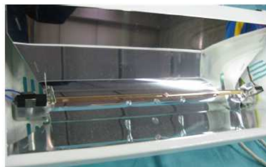
7. REINSERER LES JOINTS SILICONIQUES DANS LES DEUX RESSORTS COMME EN ORIGINE
